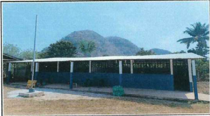
Foto 2: Se observa hundimiento en láminas y capotes debido a la mala instalación de estructura de soporte de madera, el material se dobló.
